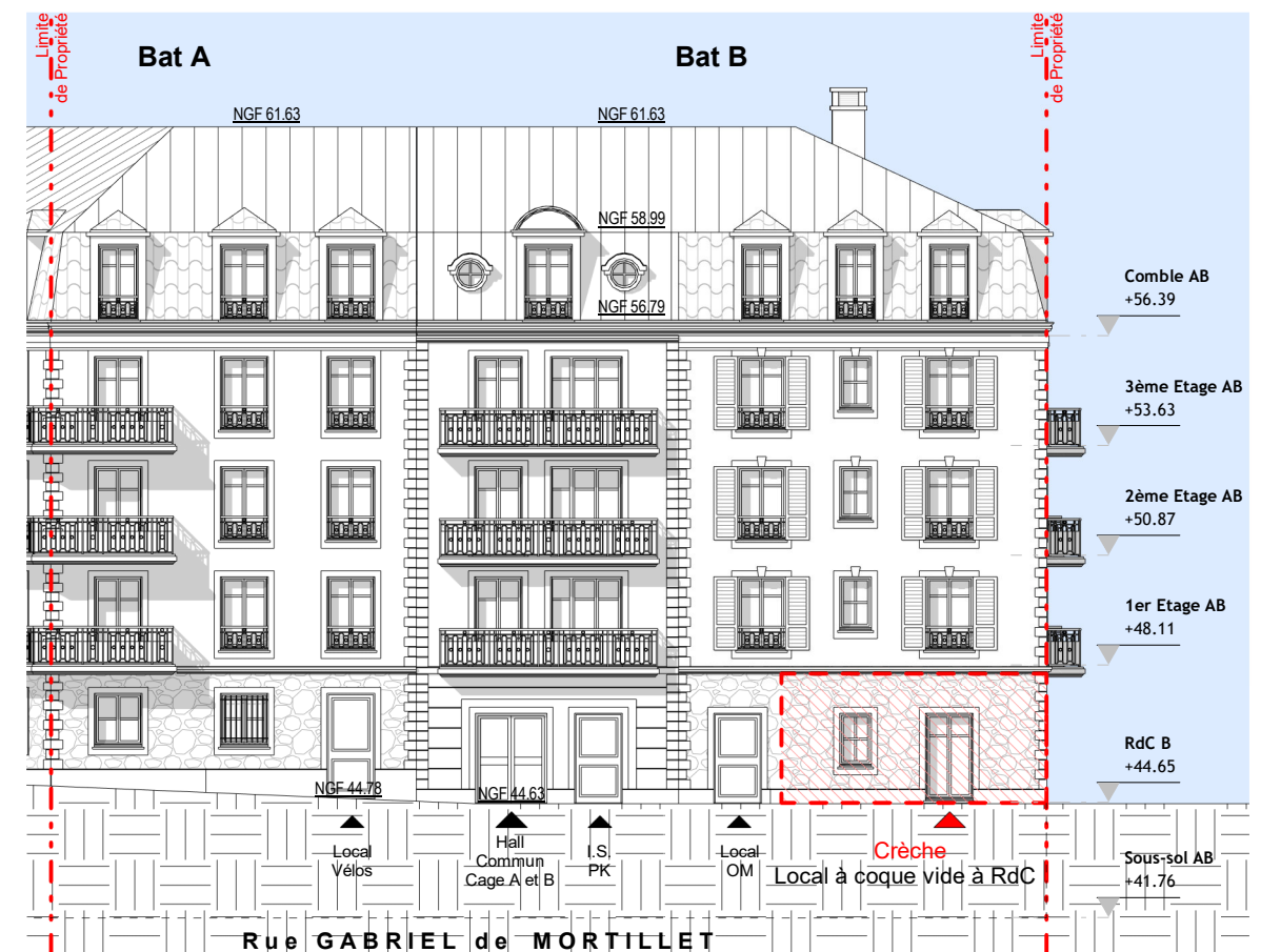
Elévation Nord-Ouest
